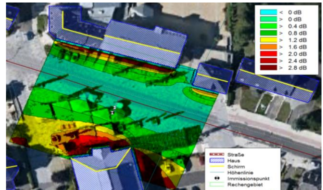
Abbildung 6: Draufsicht auf die Situation aus Abbildung 4 und 5 inkl. Mikrofonposition für die SPB-Messung.
